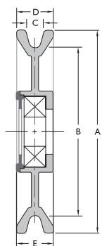
Cable Pulley
