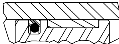
Optional Hi Load Piston
