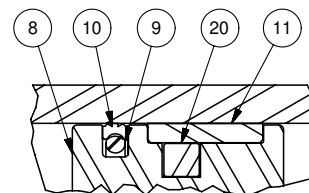
Optional Magnetic Piston
